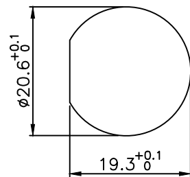
面板开孔尺寸
